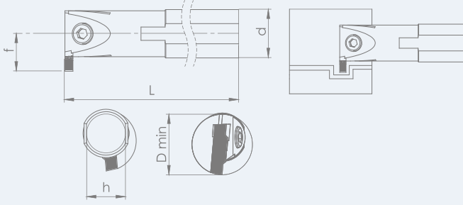
TEKNİK ÇİZİM / TECHNICAL DRAWING HORN UCUNA UYGUNDUR
