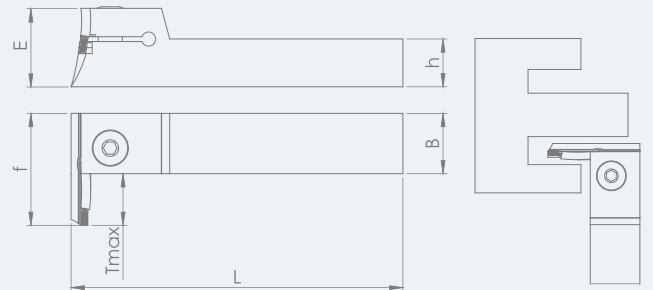
TEKNİK ÇİZİM / TECHNICAL DRAWING WALTER ÜÇUNA UYGUNDUR
