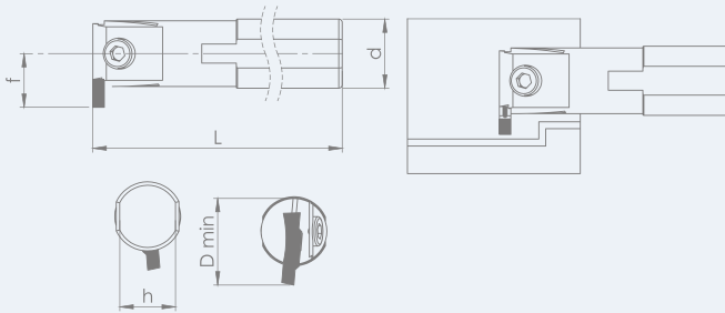
TEKNİK ÇİZİM / TECHNICAL DRAWING ISCAR UCUNA UYGUNDUR
